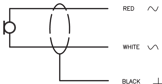
Schéma zapojení
