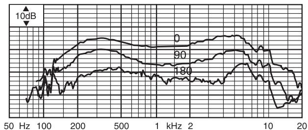
Kmitočtová charakteristika
